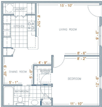
1 BEDROOM FLAT 700sq.ft.
